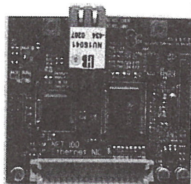
100Mb ethernet NIC Simtec
